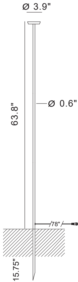
PIN MAXI - H3731-1600
