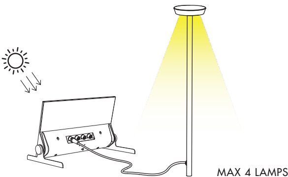
PIN MAXI - H3731-1600
