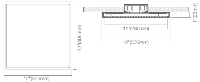
ADS12S-Tunable-5CCTYY
