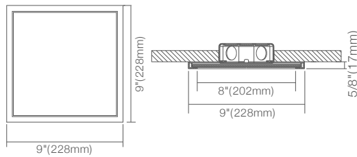
ADS9S-Tunable-5CCTYY
