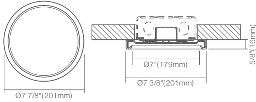
ADS7R-Tunable-5CCTYY
