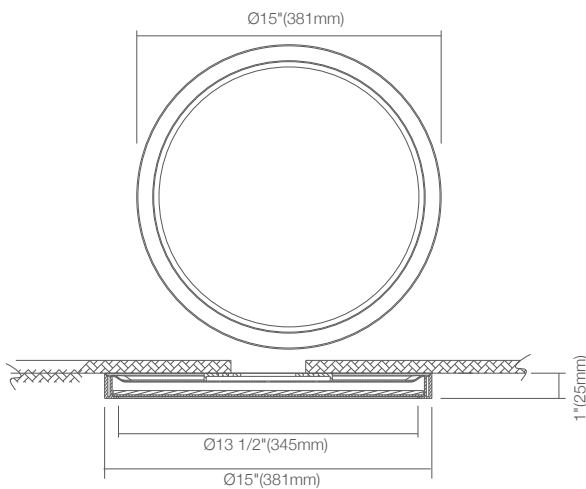
ADS15R-Tunable-5CCTYY
