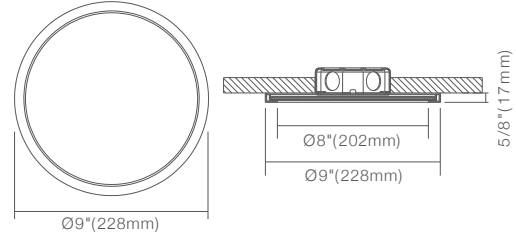
ADS9R-Tunable-5CCTYY
