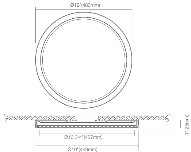
ADS19R-Tunable-5CCTYY
