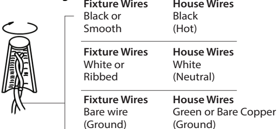
FIG. 2 Wiring
