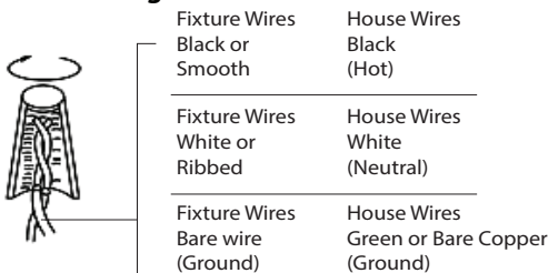
FIG. 2 Wiring
