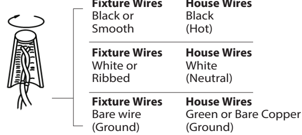
Fig. 2 Wiring
