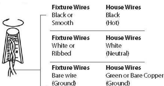
Fig. 2 Wiring
