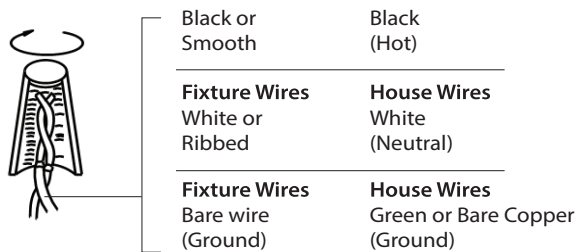
Fig. 2 Wiring
