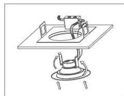
Poussez les clips vers le haut et installez-les dans l'appareil
