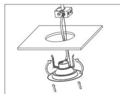
Poussez les clips vers le haut et installez-les dans l'ouverture
