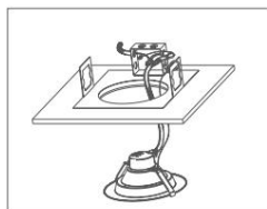
Contourner le ballast et le fil vers la j-box
