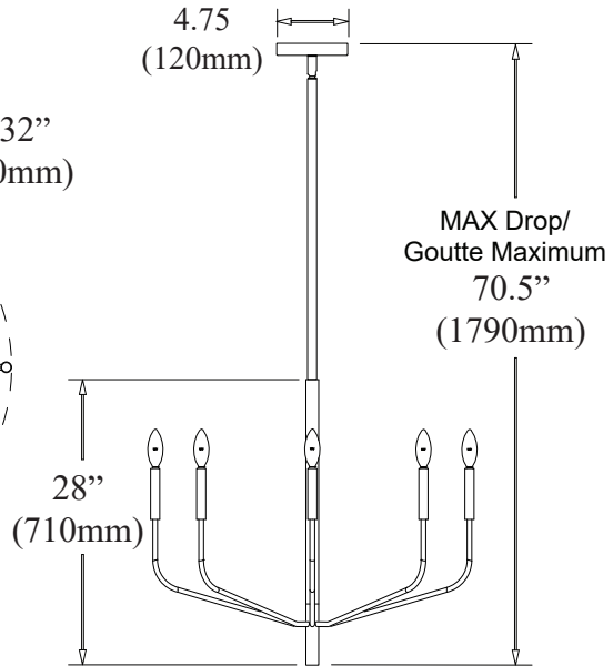
Front view Vue de face
