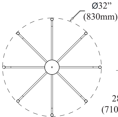
Top view Vue de dessus
